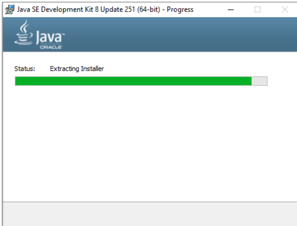
Figura 5. Instalando java.
